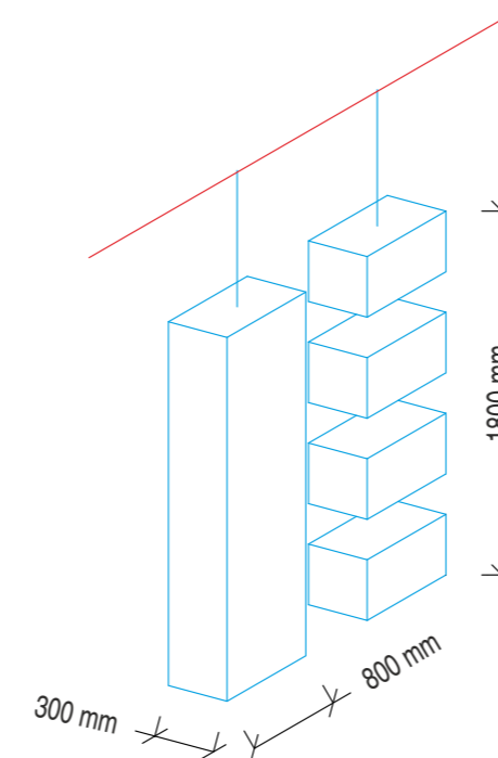
Schemat technologii wieszania detali
